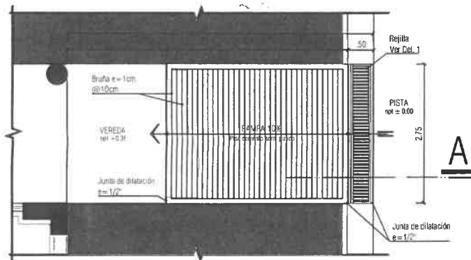
PLANO DE RAMPA Esc. 1/50
