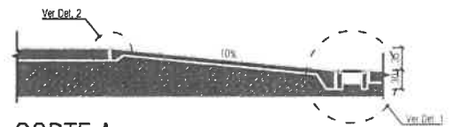
CORTE A Esc. 1/50
