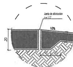
DETALLE 2 Esc. 1/10
