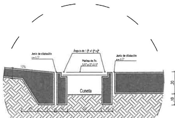
DETALLE 1 Esc. 1/10
