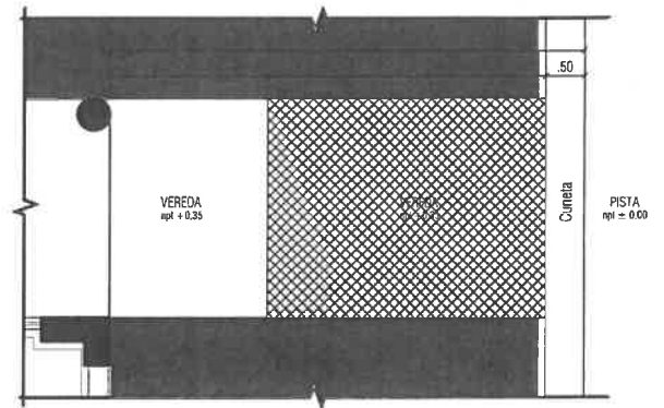
PLANO DE DEMOLICIÓN Esc. 1/50
